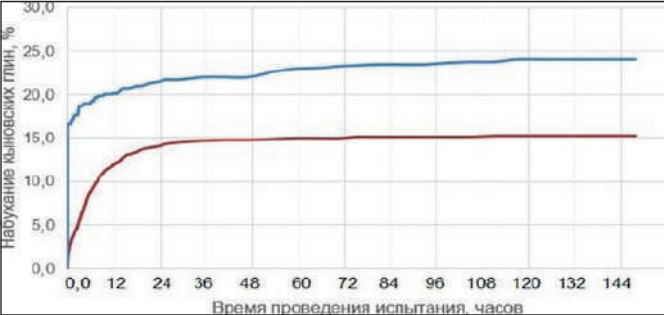
График набухания кыновских аргиллитов со временем в растворе «ГИБР-3»
